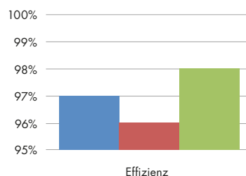
Vergleich der typischen Effizienz beim Optidrive Eco HLK und anderen AC-Frequenzumrichtern
